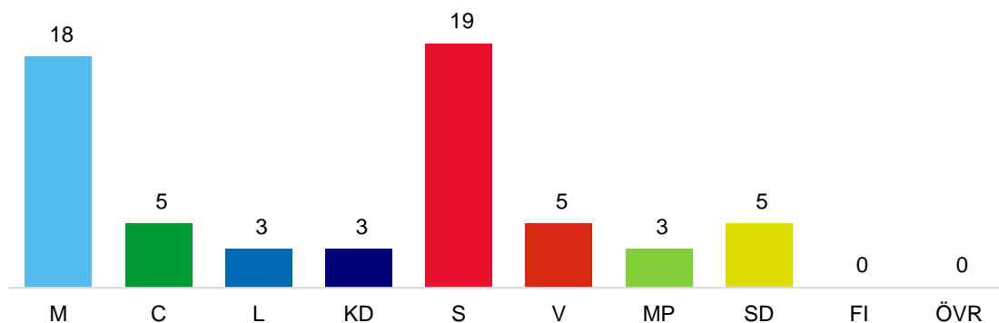
Figur 27 - Mandatfördelning i kommunfullmäktige, kommunval Växjö kommun 2018
