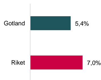
Figur 20 - Ungdomsarbetslöshet
