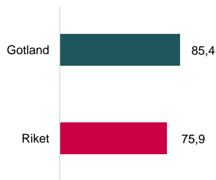
Figur 14 - Demografisk försörjningskvot, 2018
